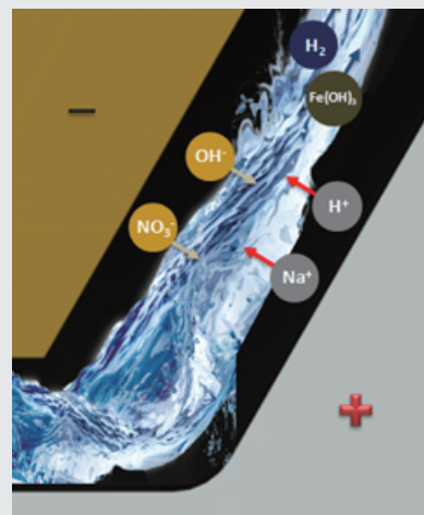
電化學加工示意圖 Electrochemical Processing Schematic
